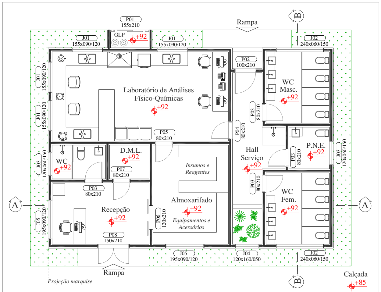
Figura 01 – Planta baixa do edifício-alvo
